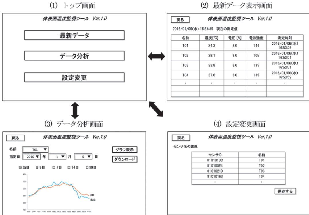
図20 各種端末のWebブラウザ画面
