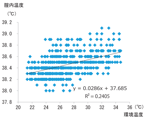
図1 環境温度と腔内温度との関係
