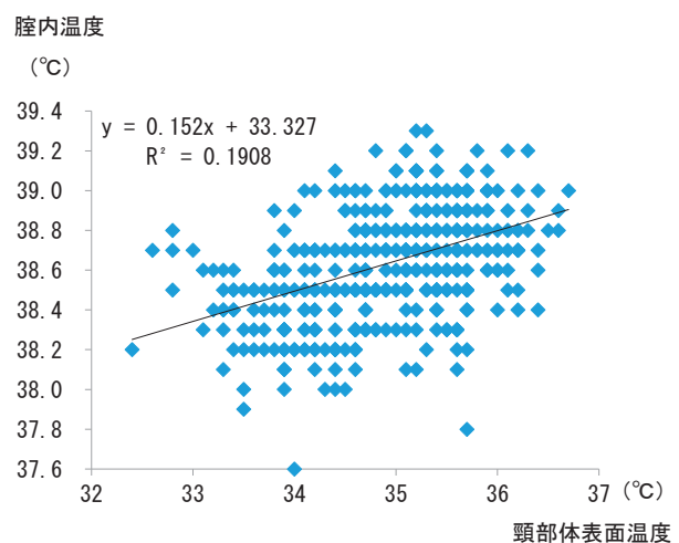
図5 頸部体表面温度と腔内温度との関係
