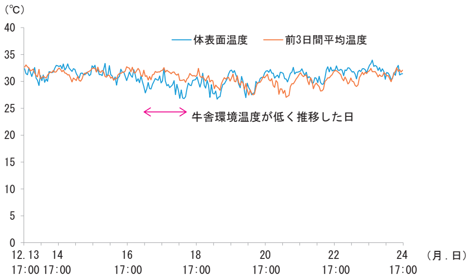
図13 肥育牛における頸部体表面温度の推移 (No.T1)
