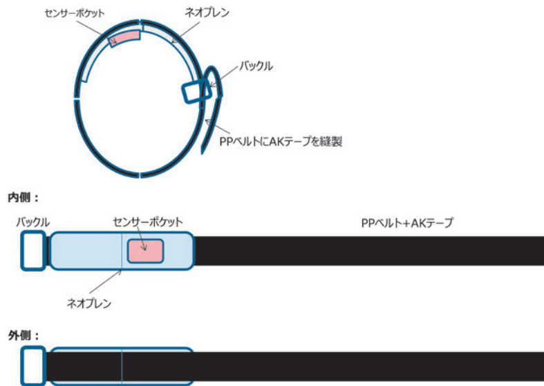
図7 ウェアラブルネックベルト
