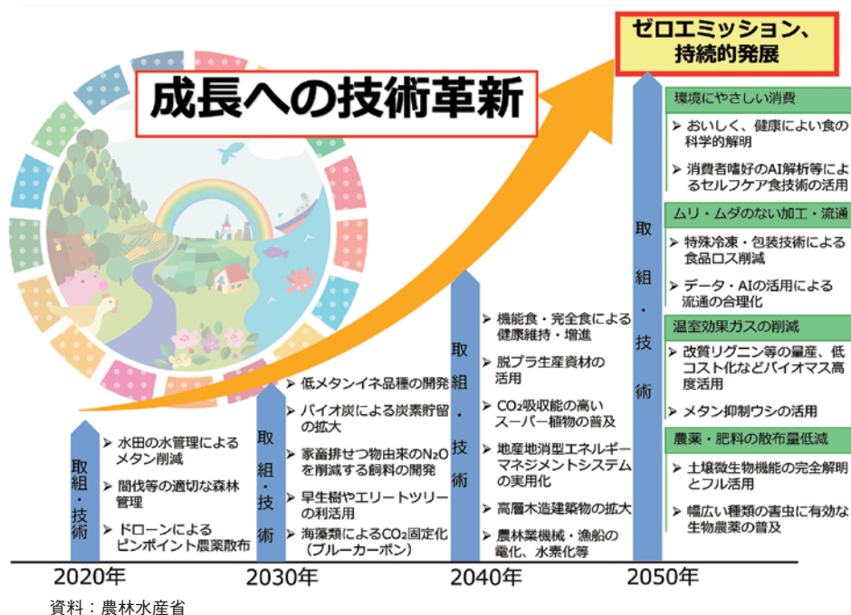
図5 農林水産分野でのゼロエミッション達成と持続的発展に向けた取組
