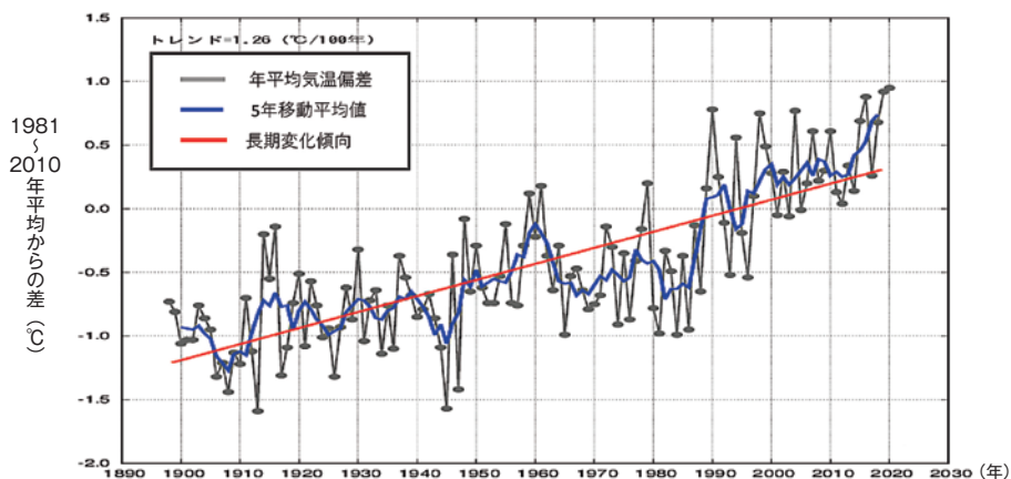
図1 日本の年平均気温偏差（気候変動監視レポート2020）
